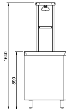
End Elevation
