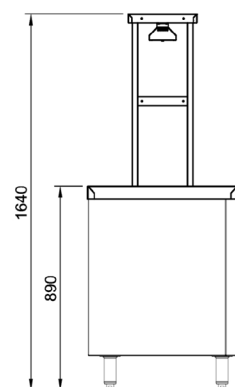
End Elevation
