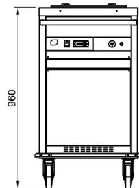
End Elevation
