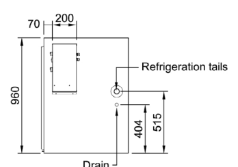
End Elevation
