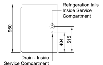
End Elevation
