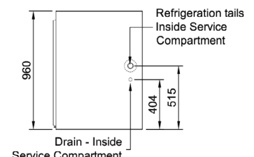
End Elevation
