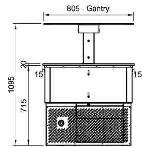
End Elevation
