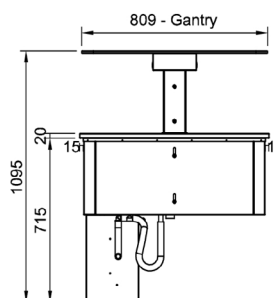
End Elevation
