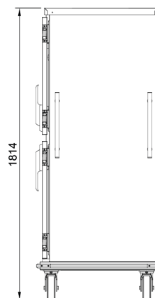
End Elevation
