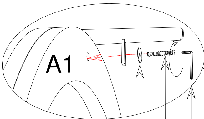
DETAIL: 2.1
