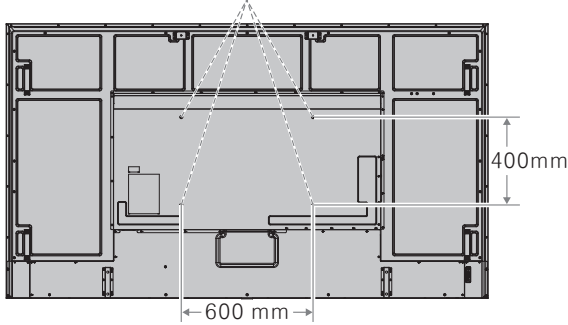
마운트 인터페이스(M8)
