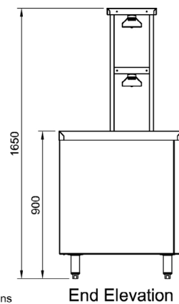
End Elevation
