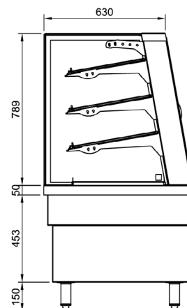
End Elevation
