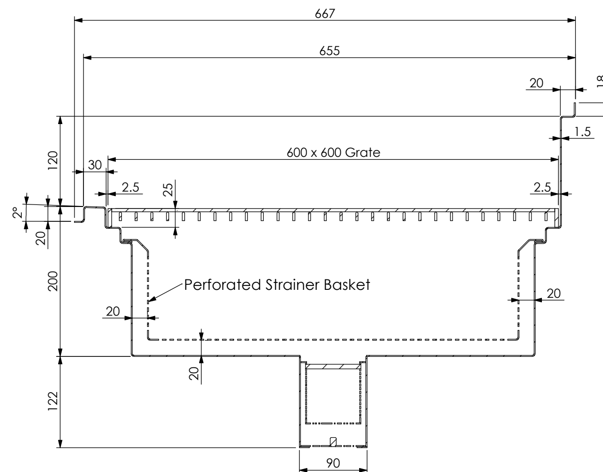
SECTION A-A SCALE 1 : 5
