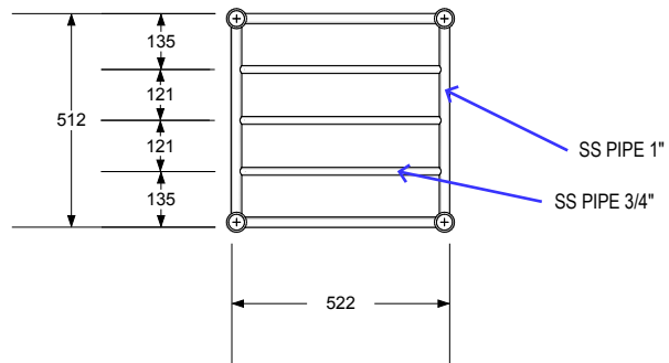
TOP ELEVATION
