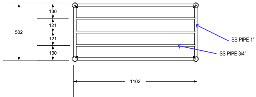
TOP ELEVATION
