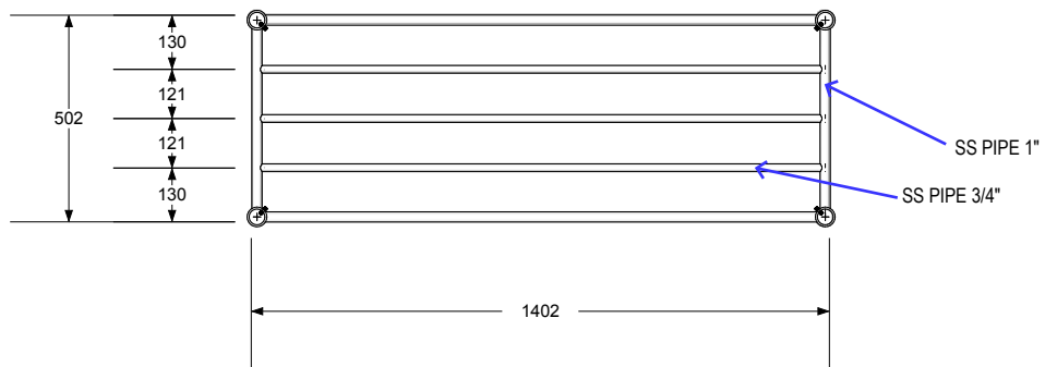
TOP ELEVATION
