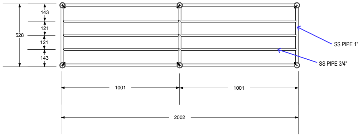
TOP ELEVATION
