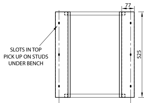
TOP ELEVATION
