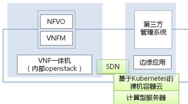
图 8 裸机容器云
