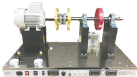
MVS-520 Vibrasjon og oppretting
