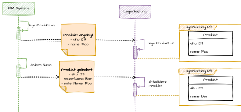
Abbildung 6.3: Ein Produkt wird in einem PIM System erstellt und aktualisiert, während ein Lagerhaltungssystem eine nachlaufende Kopie dieser Daten hält
