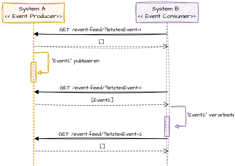
Abbildung 6.1: Ein Konsument ruft Events über eine HTTP-Feed-Schnittstelle des Produzenten ab.
