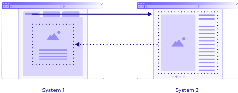
Abbildung 5.2: UI Elemente eines anderen SCS werden integriert
