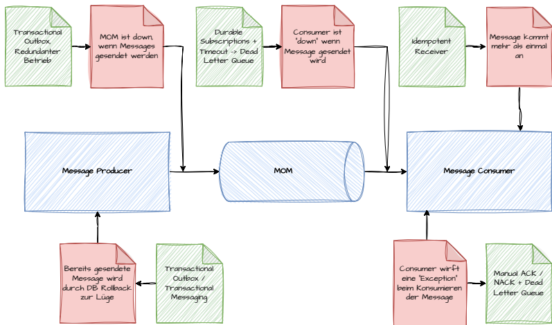
Abbildung 6.5: Übersicht gängiger Risiken (rote Klebezettel) beim Messaging sowie gängiger Lösungen (grüne Klebezettel) für diese Probleme.
