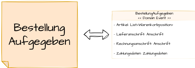
Abbildung 6.2: Ein Domain Event als Klassendiagramm mit dem entsprechenden orangenen Post-it
