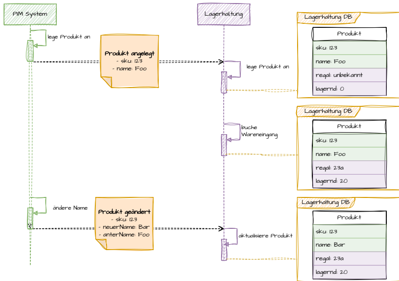
Abbildung 6.4: Unser repliziertes Produkt wird mit eigenen fachlichen Attributen „angereichert“
