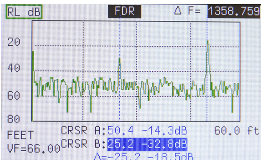
FDR
