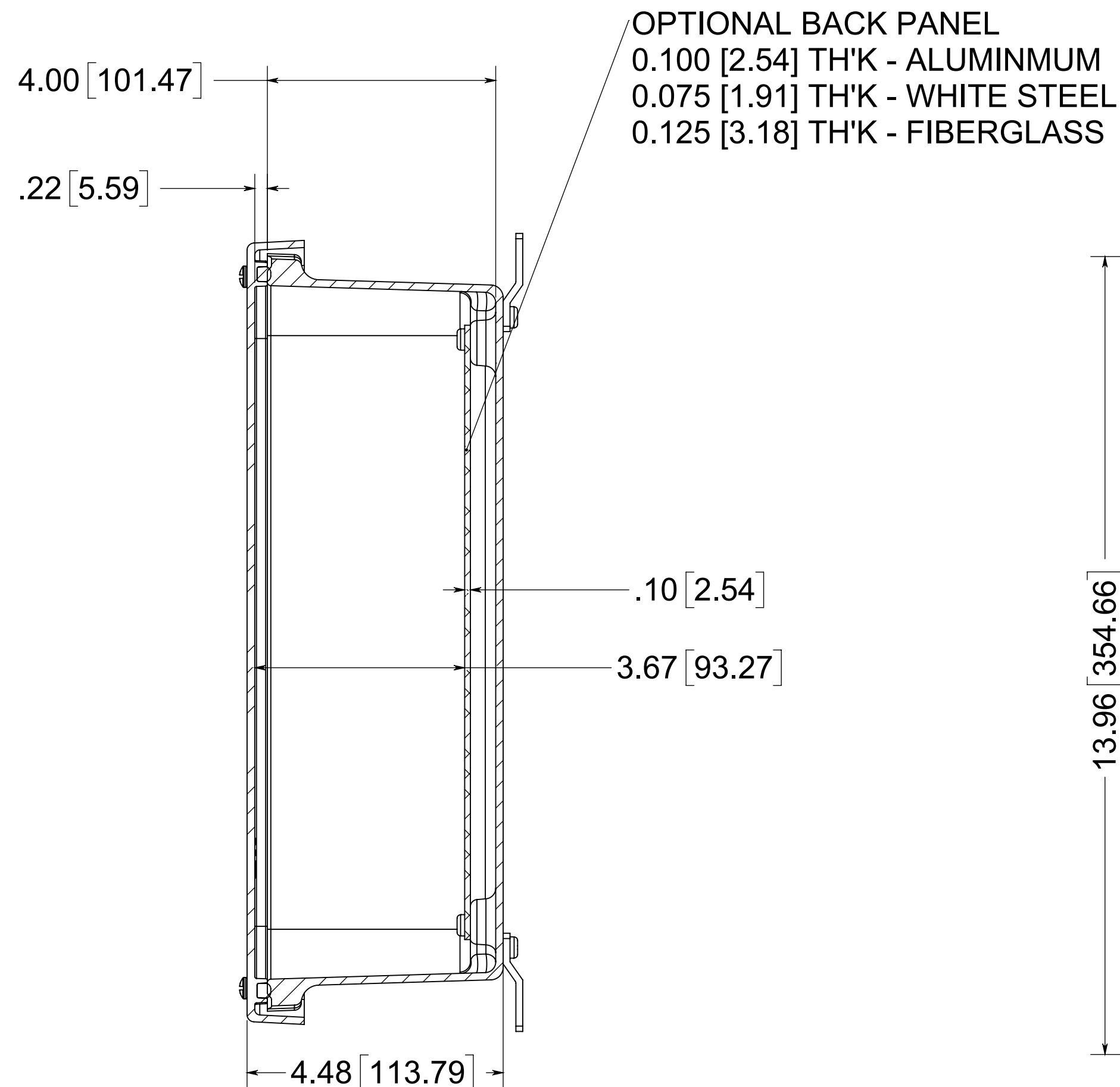
SECTION A-A
