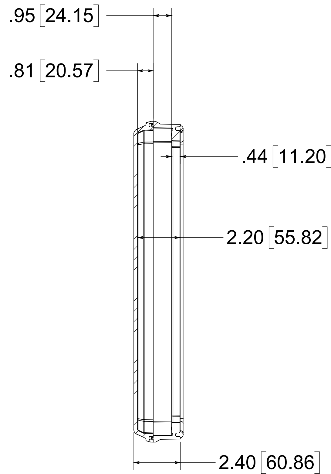
SECTION A-A
