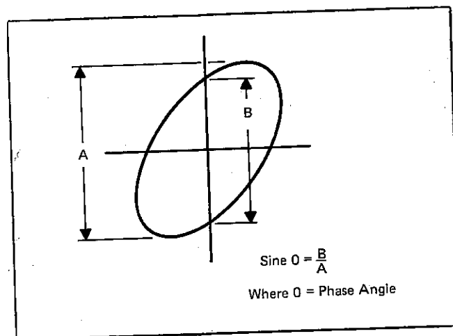
Fig. 26. Phase shift calculation.
