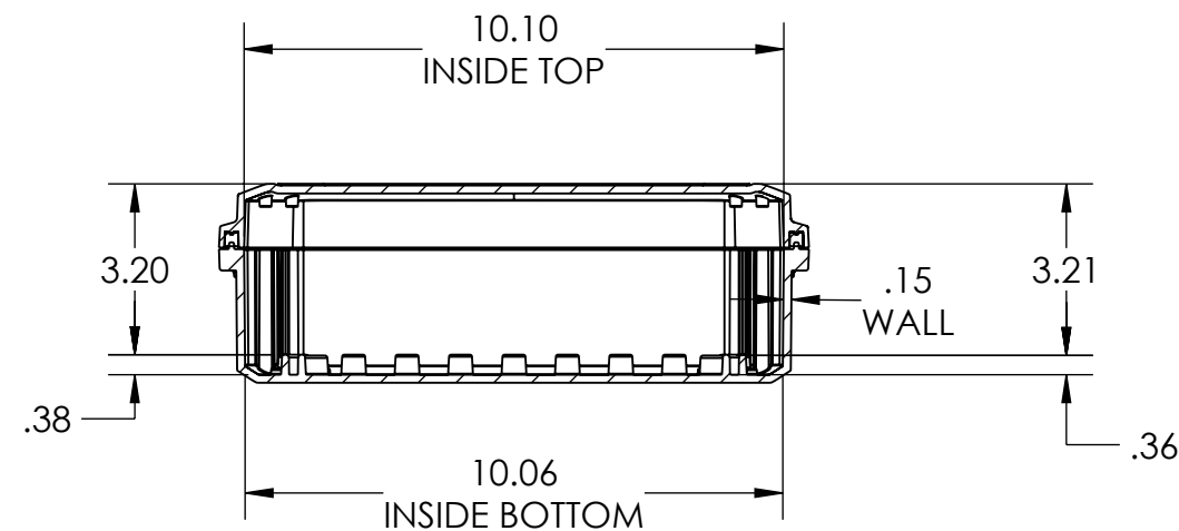
SECTION A-A SCALE 1 : 4
