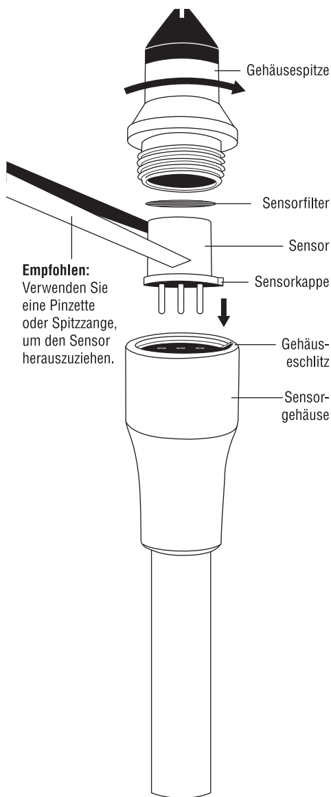
Abbildung: Sensoraustausch
