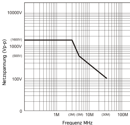
Figure 4. Derating/ herabgestufte Spannungskurve
