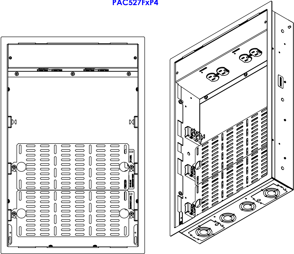
PAC527FxP4
