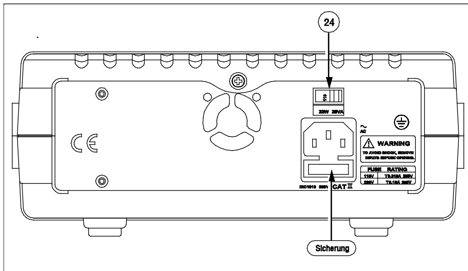
Fig. 2 FG2C-UA Rückseite
