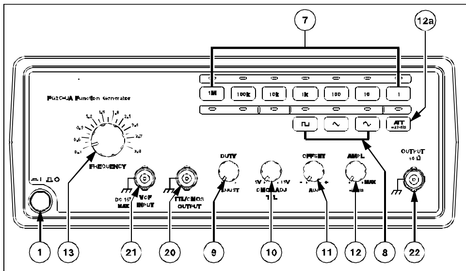
Fig. 1 FG2C-UA Frontansicht
