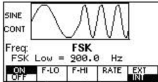
FSK Menu
