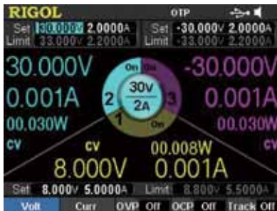
DP831A GUI
