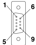
CN-2 (D-Sub 9-pin side)
