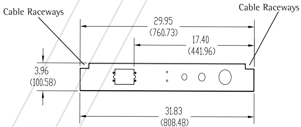
INW-AM325 (top view)
