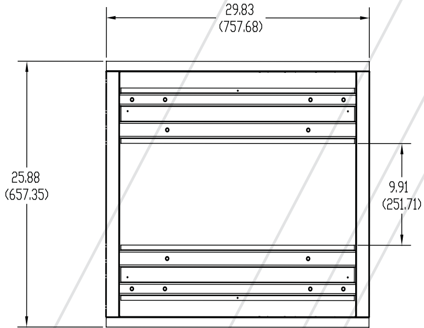
INW-AM325 (front view)
