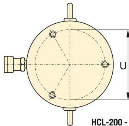
HCL-50 - 150 ton
