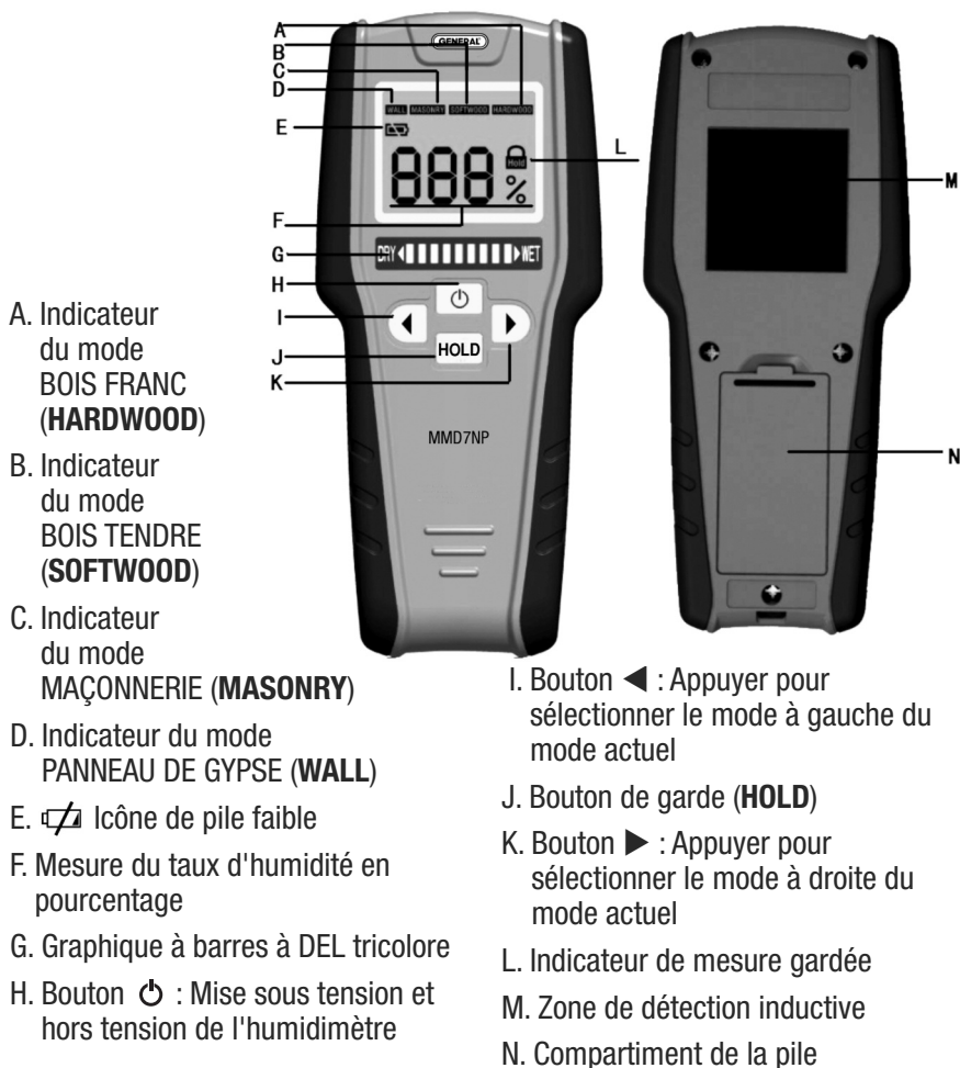
Fig. 1 Touches, indicateurs et caractéristiques physiques du MMD7NP
