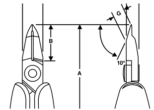
RX8233A, RX8234A
