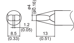
TX2-XBCR6 Shape-6XBCR
