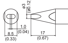
TX2-XBCR4 Shape-4XBCR
