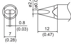
TX1-XBCR4 Shape-4XBCR
