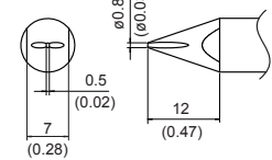
TX1-XBCR2 Shape-2XBCR
