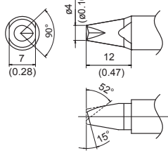
TX1-XDR3 Shape-3XDR
