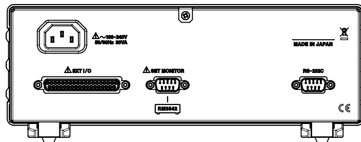
背面図
