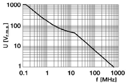
Figura 1-12 Sonda 10:1 - oscilloscopio U1561A
