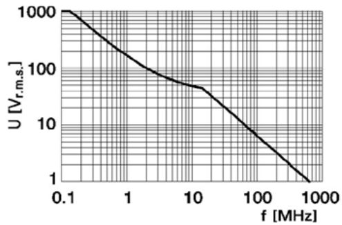
Figure 1-12 U1561A avec sonde 10:1
