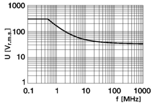
Figura 1-11 Sonda 1:1 - oscilloscopio U1560A
