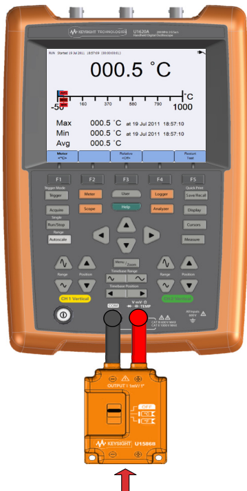
Sonda termopar tipo K
