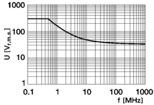
Figure 1-11 U1560A avec sonde 1:1
