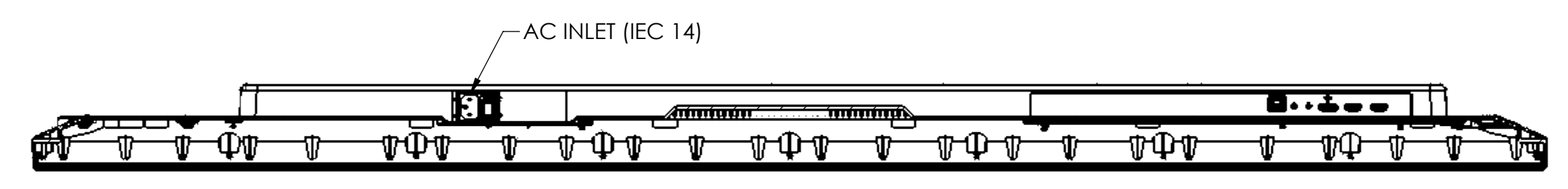
SECTION A-A
