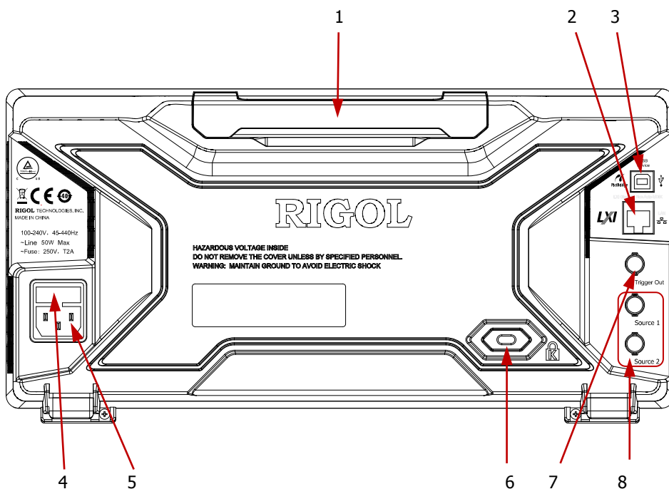
图 11 后面板总览
