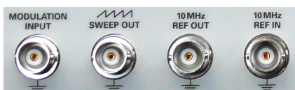
Abb. 7.3: Anschlüsse an der Geräterückseite
