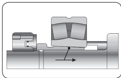
Bild 13. Zwei Gleitflächen
