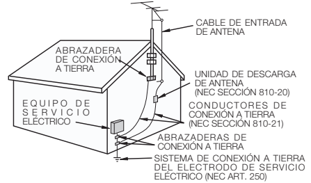
EJEMPLO DE CONEXIÓN A TIERRA DE LA ANTENA SEGÚN EL CÓDIGO ELÉCTRICO NACIONAL, ANSI/NFPA 70
