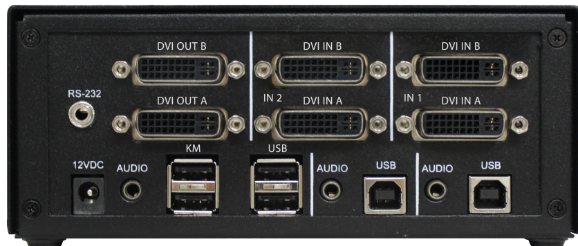
SM-DVN-2D Back
