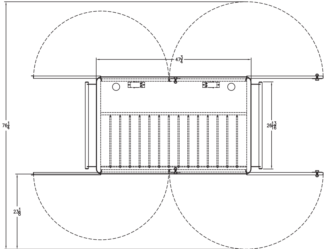
vLT-30 Laptop Cart
