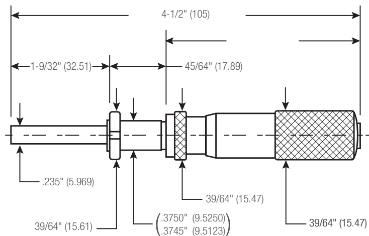
263L-38TN (0-1") dimensions
