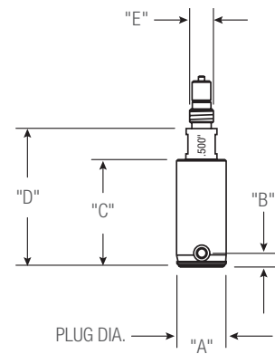
M6 AccuPlug
