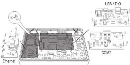
Figura 1-5: Posizioni scheda opzionale
