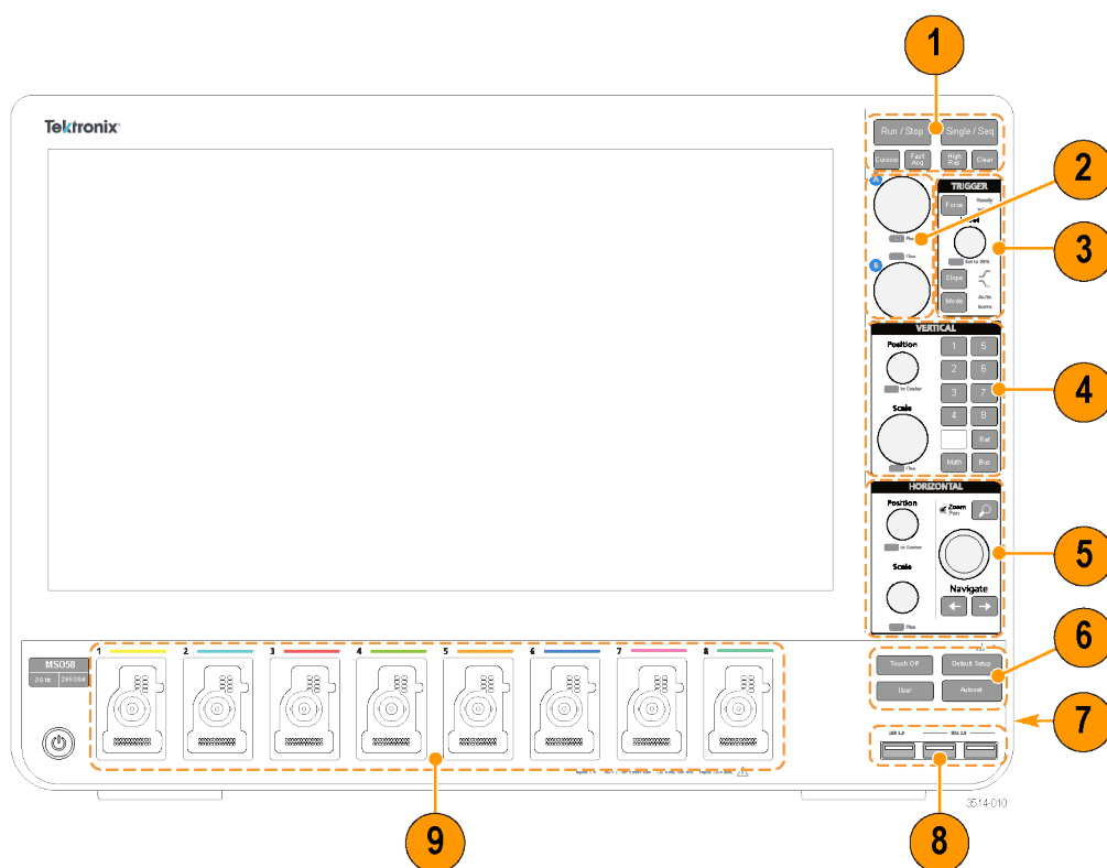
図 3 : 5 シリーズ MSO のコントロール
