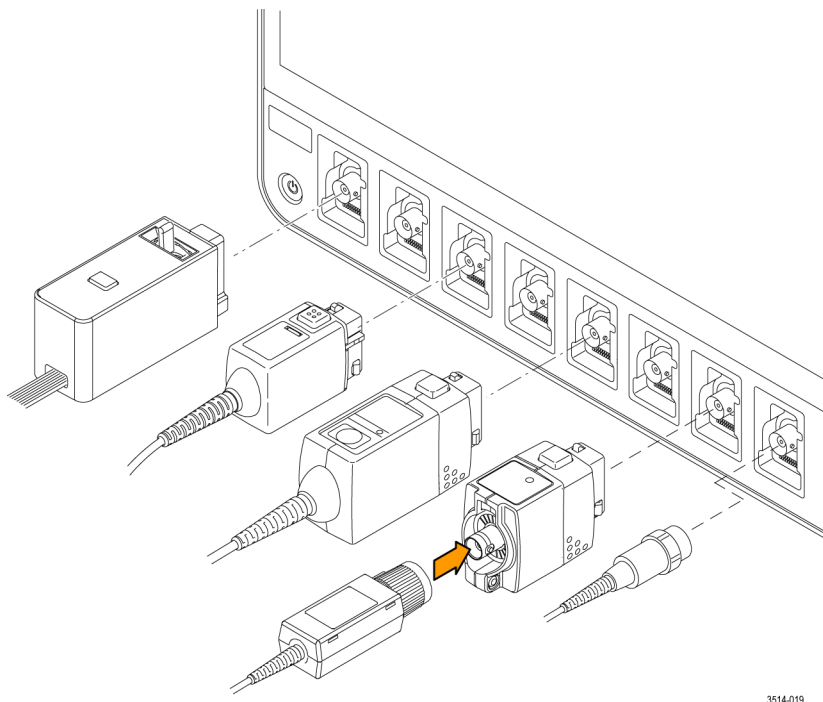
图 2: 将探头连接 MSO54、MSO56 或 MSO58
