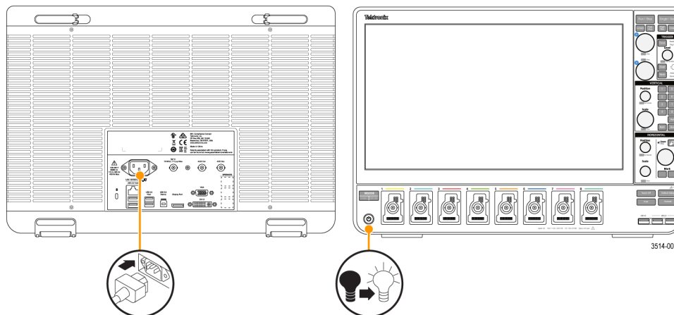
図 1 : MS054 型、MS056 型、MS058 型の電源コード・コネクタと電源スタンバイ・スイッチ
