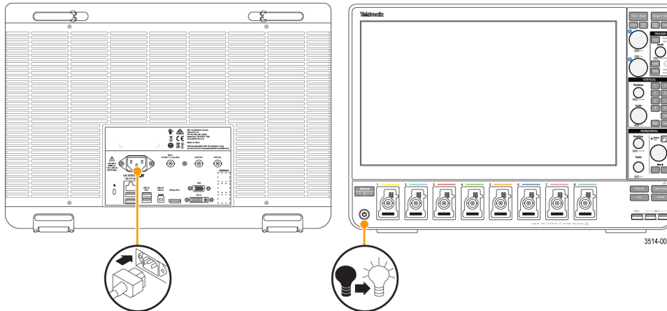
图 1: MS054、MS056、MS058 电源线连接器和电源待机开关
