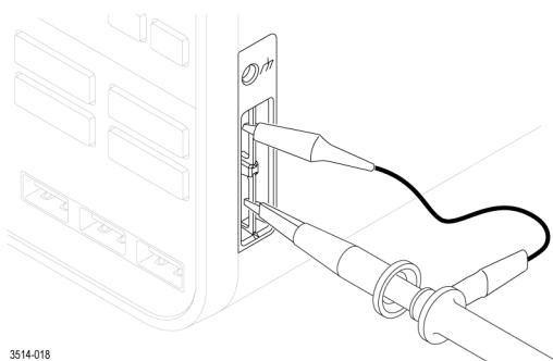
图 4: 5 系列 MSO 仪器上的探头补偿连接器。
