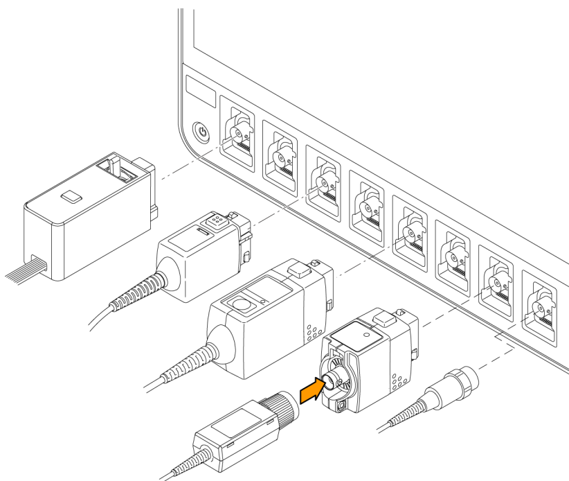
図 2：MSO54 型、MSO56 型、または MSO58 型へのプローブの接続
