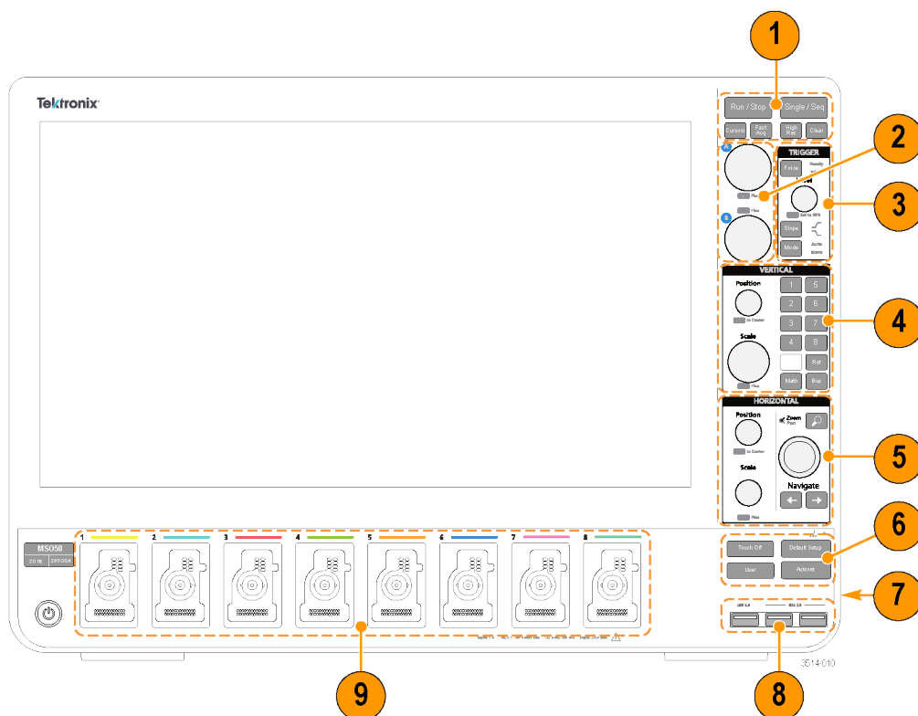
图 3: 5 系列 MSO 控件
