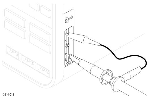
図 4:5 シリーズ MSO でのプローブ補正の接続
