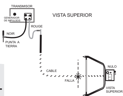
Figura 5. Receptor de Anulación - Segunda Vez
