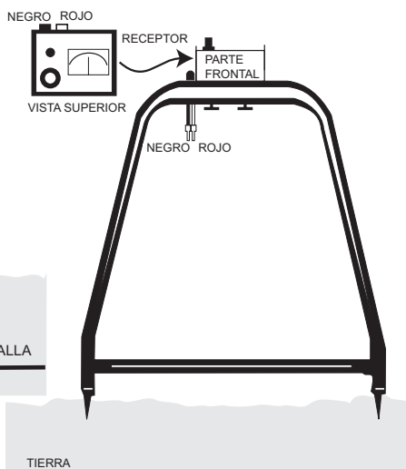
Figura 2. Instalación del Receptor
